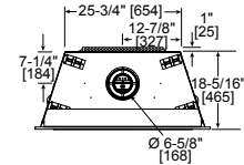
RAVE3012I Dimensions
